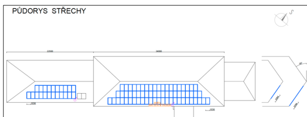
Obrázek 5 Rozmístění panelů FVE škola Sruby
